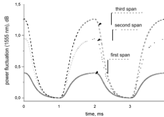
Figura 1. Distribución de potencia del canal a 1555 nm a lo largo del enlace de 383 km (Fuente: LNCS 5412, pág. 323)
